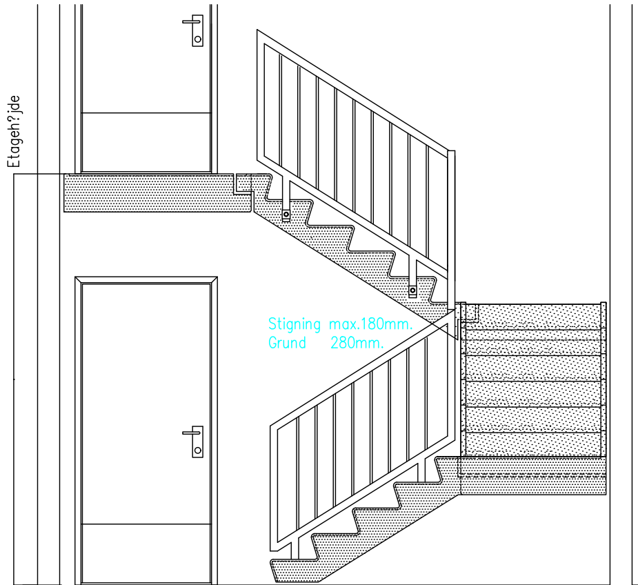
Opstalt af Trapperum
