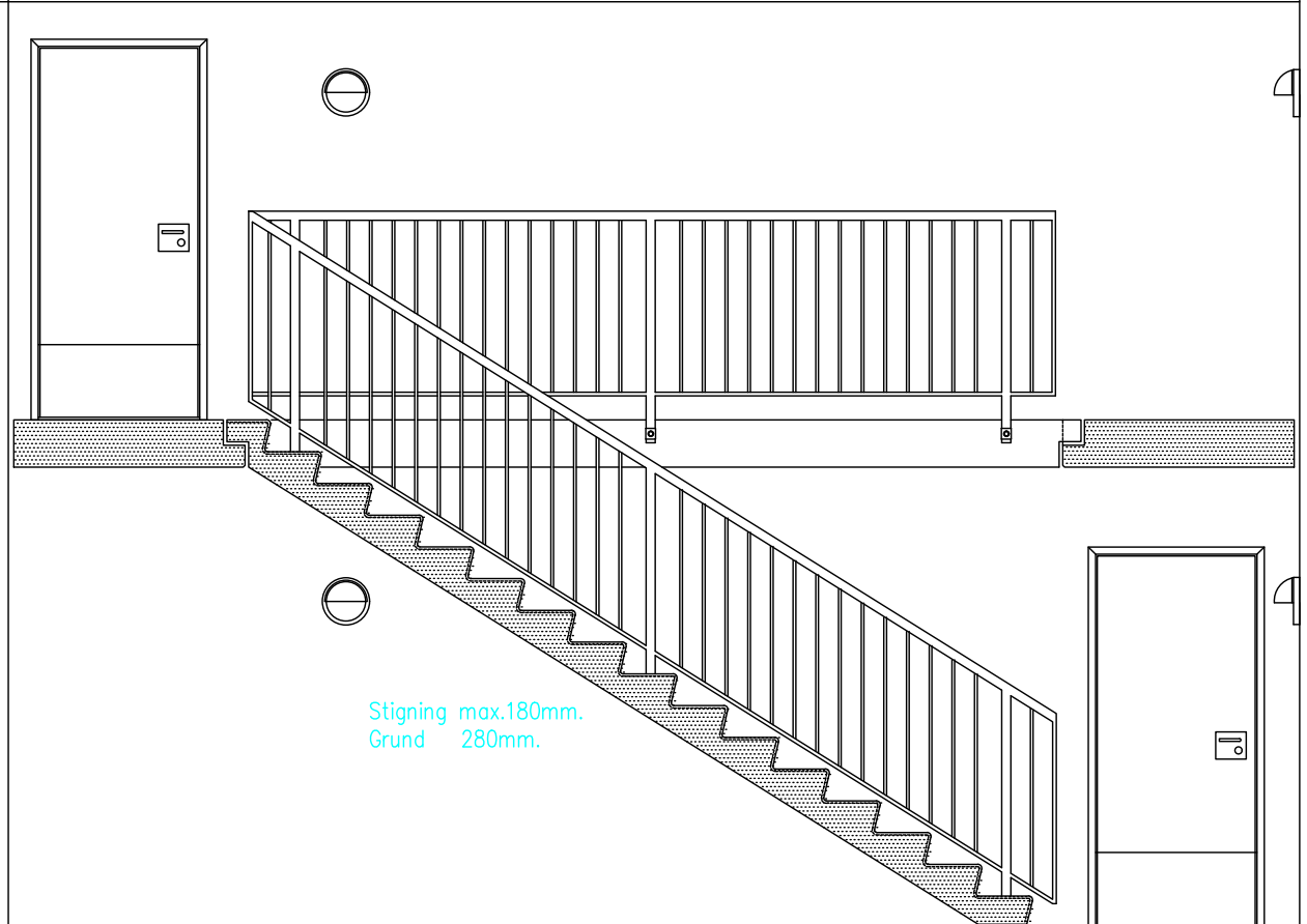
Opstalt af Trapperum
