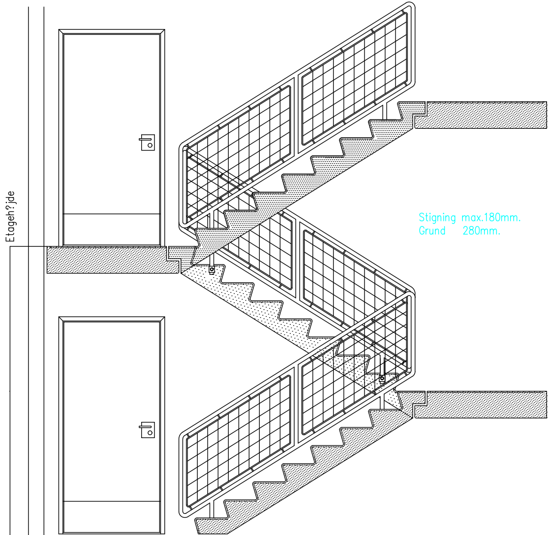
Opstalt af Trapperum
