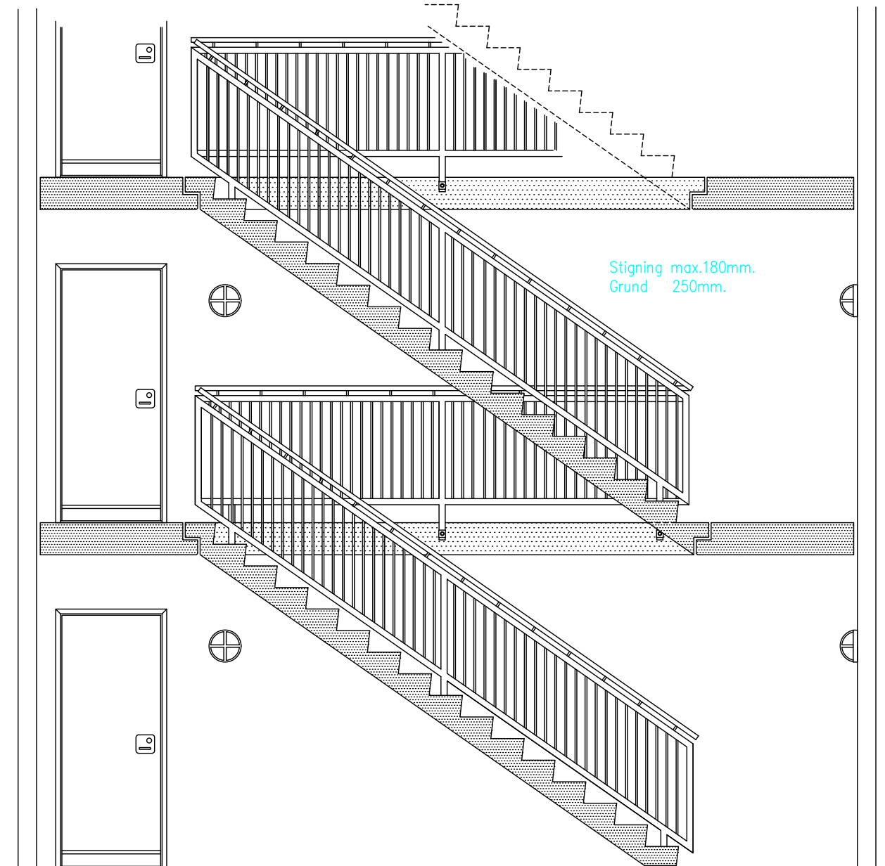
Opstalt af Trapperum
