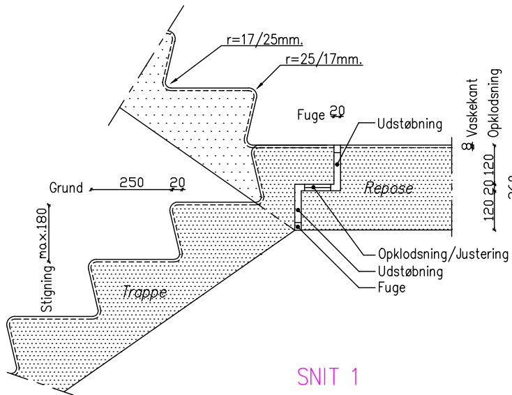
Samling med trappe og Repos.
