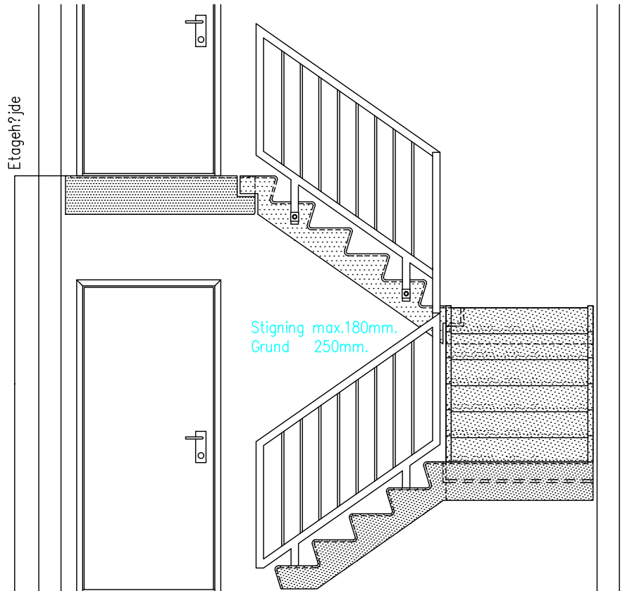
Opstalt af Trapperum
