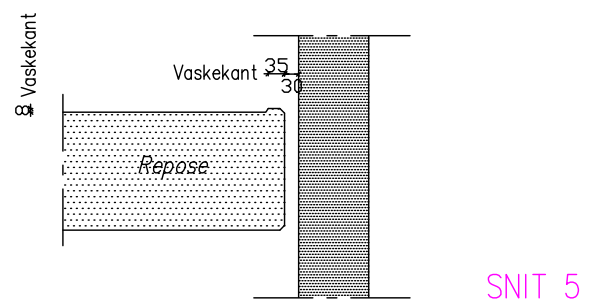
Fuge ved Trappeløb/Væg.
