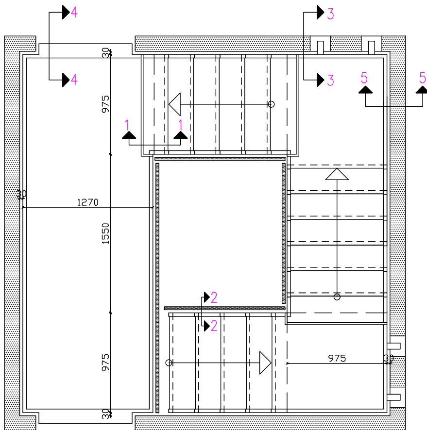
Plan af Trapperum
