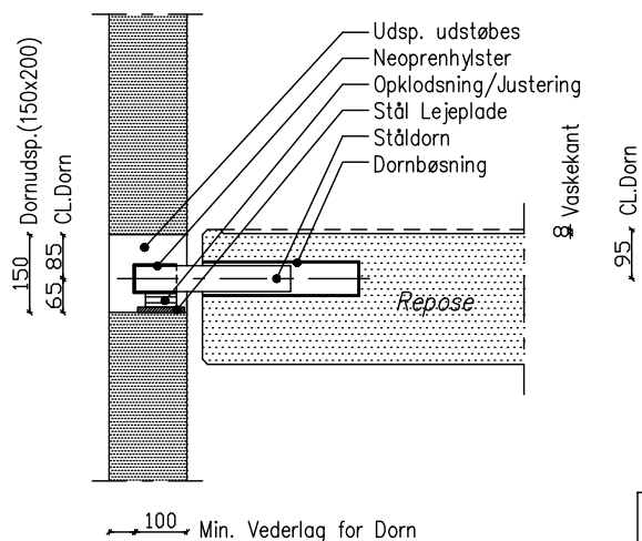
Dornsamling mellem repos og væg.
