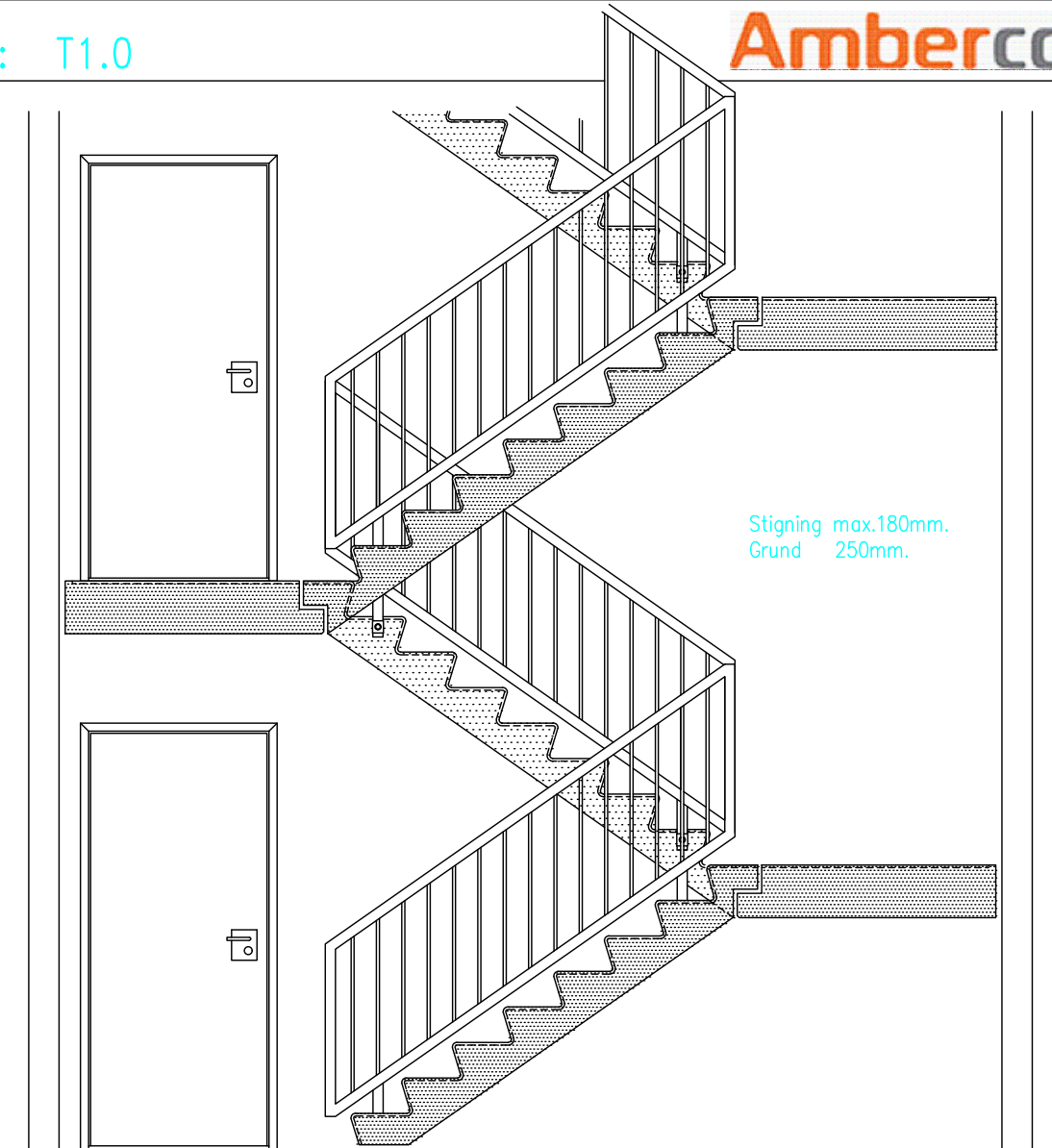
Opstalt af Trapperum
