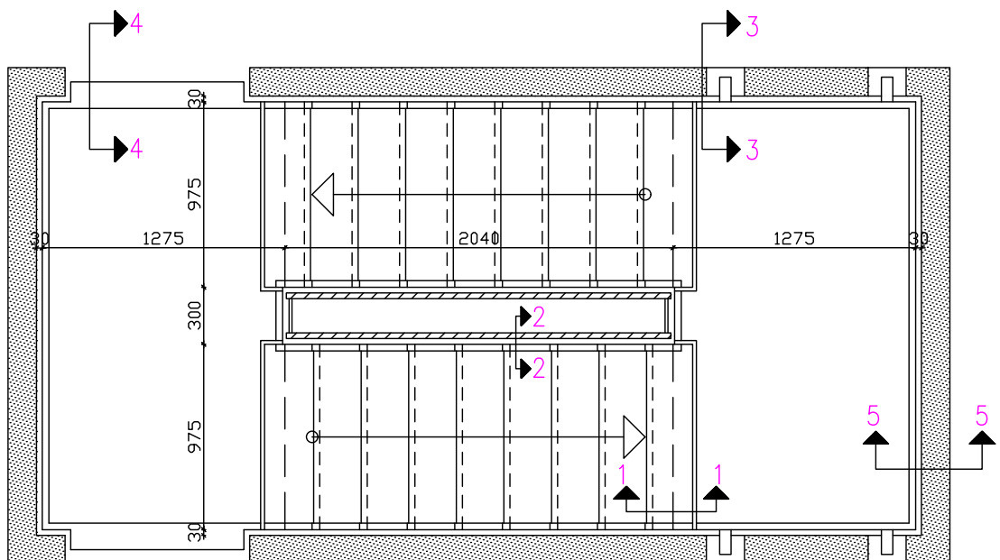
Plan af Trapperum
