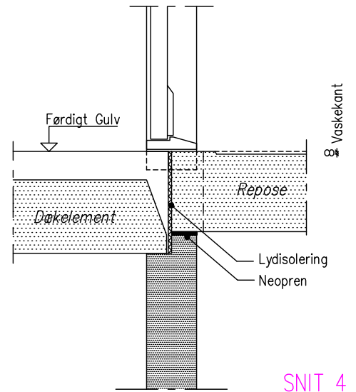
Repo vederlag i dørudsp.
