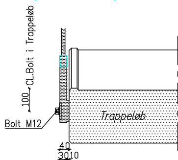
Fastgørelse af gelænder til trappeløb.
